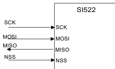
图 8.1 SPI 接口
