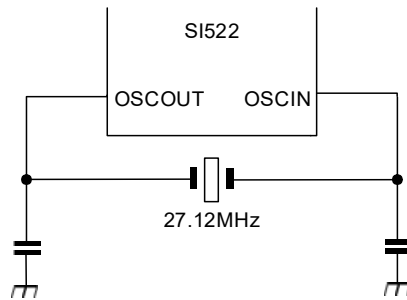
图 14.1 晶振连接
