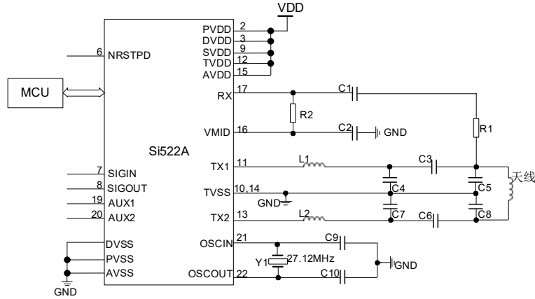
图 17.1 Si522A 典型应用电路图
