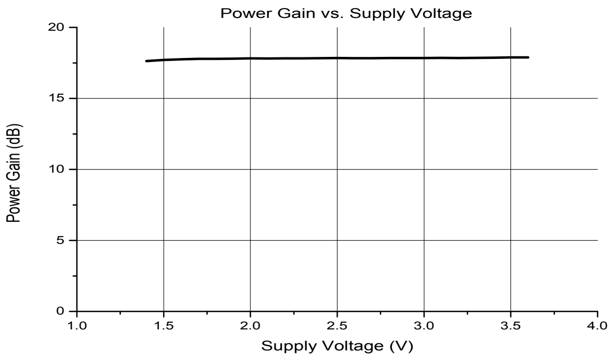
图三、功率增益与供电电压的曲线
